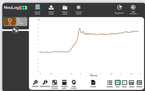
Měření třecí síly
