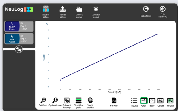
Ohmův zákon
