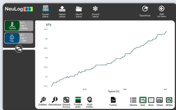
Zákon absolutní nuly – zákon Gay-Lussaca
