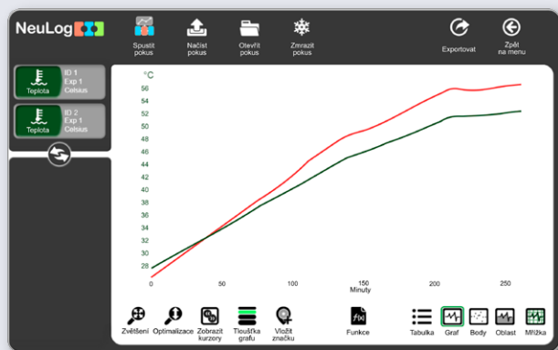
Skleníkový efekt
