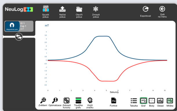
Silové působení magnetického pole
