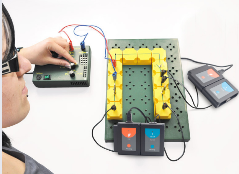
Ohmův zákon
