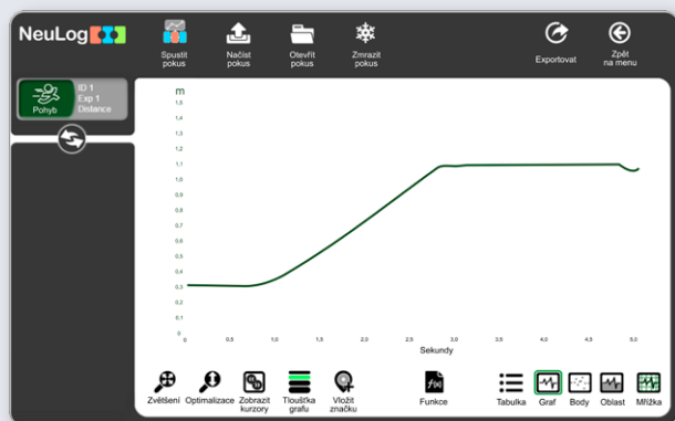
Rovnoměrný pohyb
