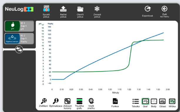
Titrace roztoku
