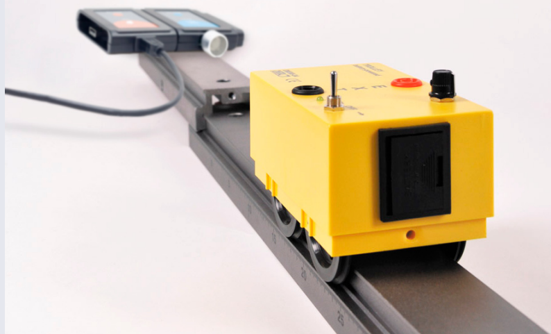
Rovnoměrný pohyb
