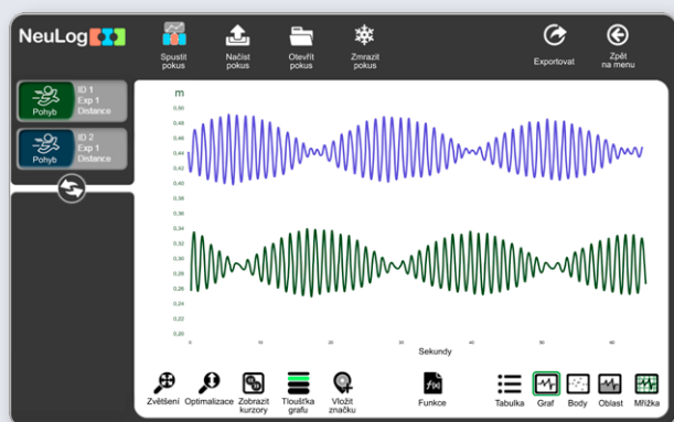
Propojené kyvadlo
