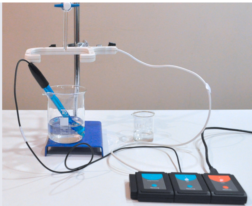
Titrace roztoku
